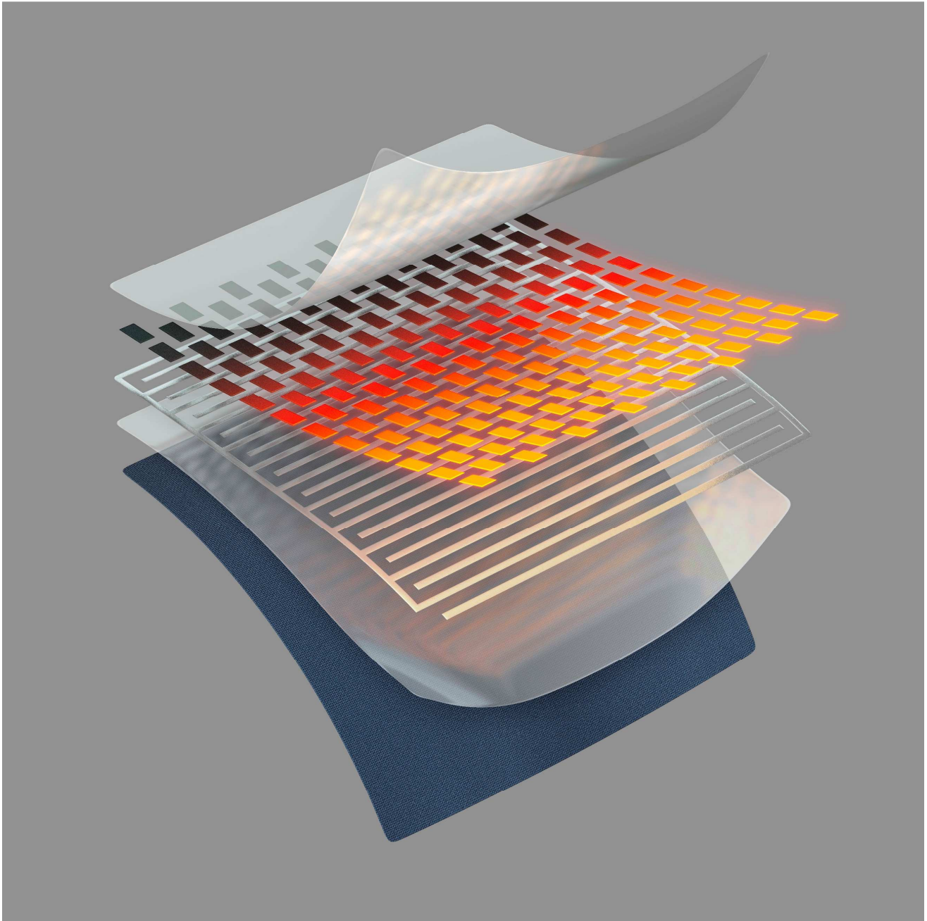
杜邦™ Intexar™ 加熱模組示意圖
